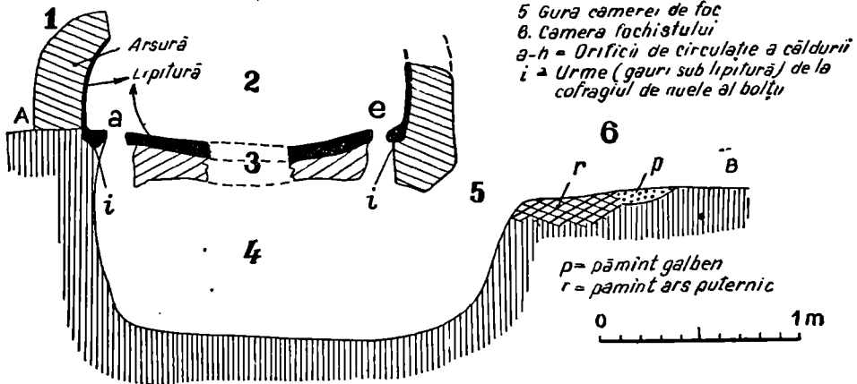
PLANȘA VIII.—Planul și profilul cuptoarelor de ars ceramică din sec. XV, descoperite la Suceava.
