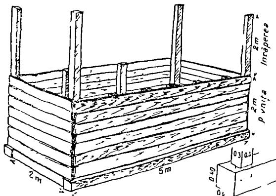
Fig. 4. — Pivnița nr. 1 (reconstituire). Schița pivniței și a îmbucării birnelor verticale cu talpa.
